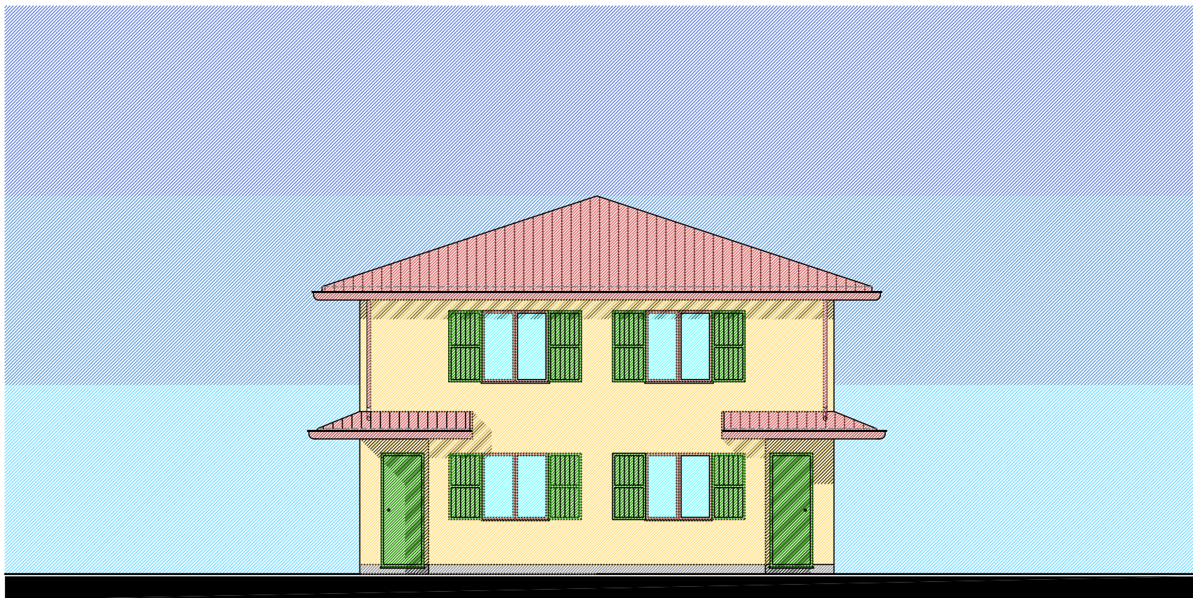
PROSPETTO NORD
